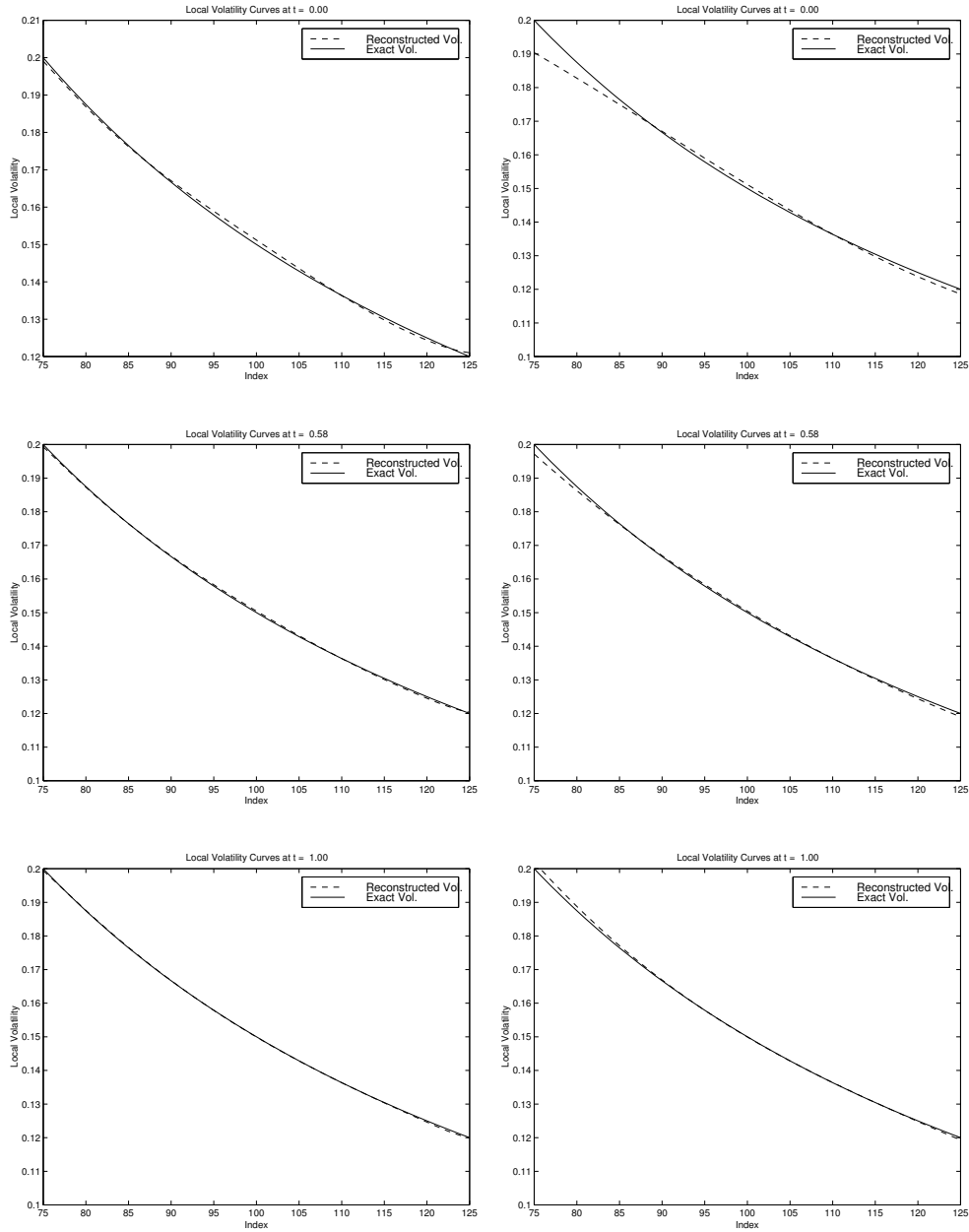
FIG. 3. Left: Knots = [0 : 20 : 200] \times [0, 1] , Right: Knots = [\cdot 4S_{\text{init}} : \cdot 4S_{\text{init}} : 1.6S_{\text{init}}] \times [0, 1]
